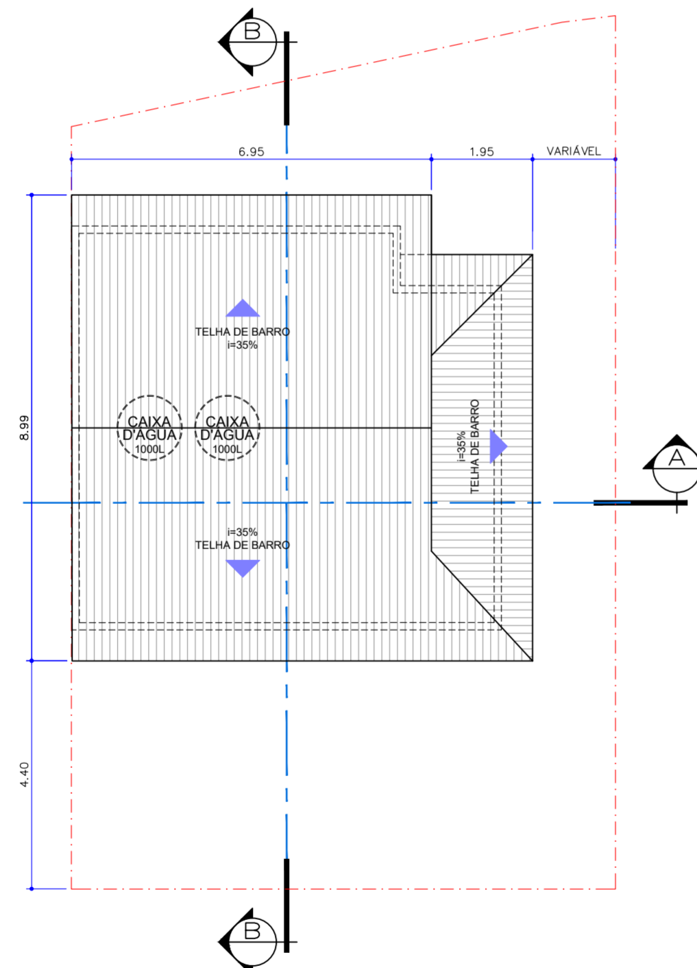
CASA TIPO C3 DIREITA (terreno em declive) PLANTA COBERTURA ESC. 1:100 MODELO IMPLANTADO EM LOTES DE GEOMETRIA IRREGULAR
