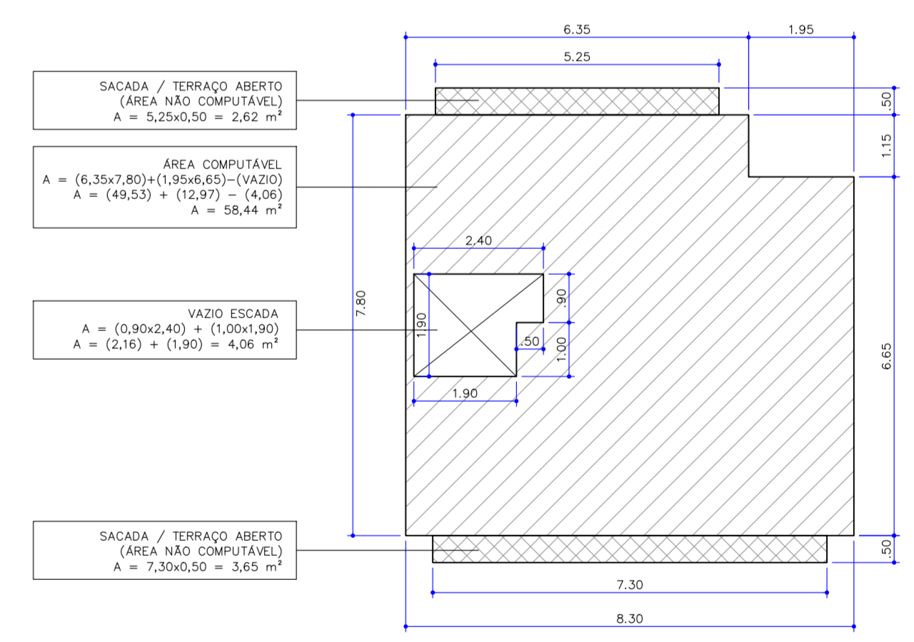
ÁREA COMPUTÁVEL = 58,44 m² ÁREA NÃO COMPUTÁVEL = 6,27 m² ÁREA TOTAL = 64,71 m² CASA TIPO C3 DIREITA PAV. INFERIOR ESC. 1:100
