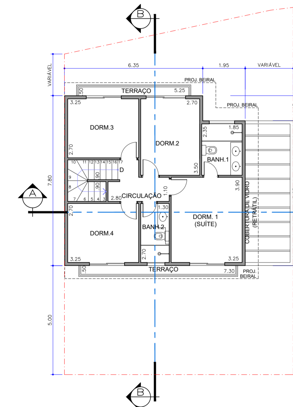
CASA TIPO C3 DIREITA (terreno em declive) PLANTA PAV. SUPERIOR ESC. 1:100 MODELO IMPLANTADO EM LOTES DE GEOMETRIA IRREGULAR
